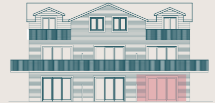
Ansicht Garten
